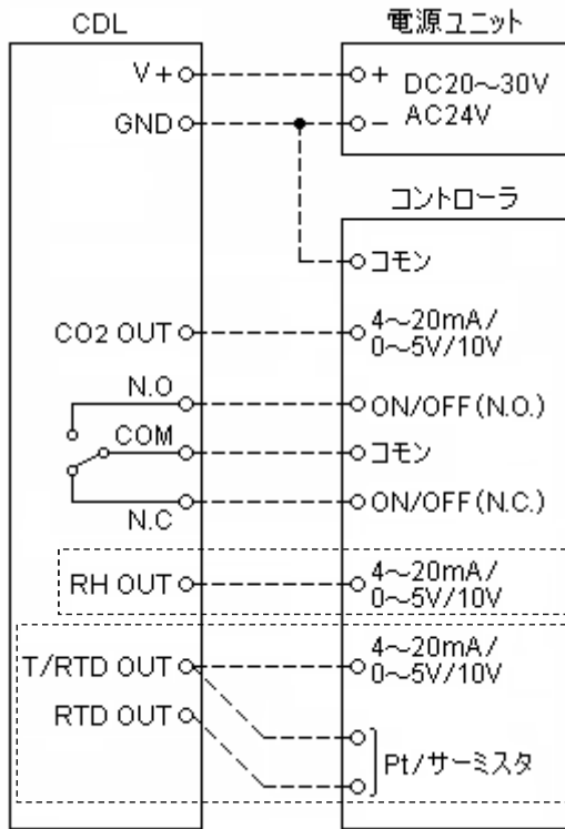
図 6. CDL 結線図
